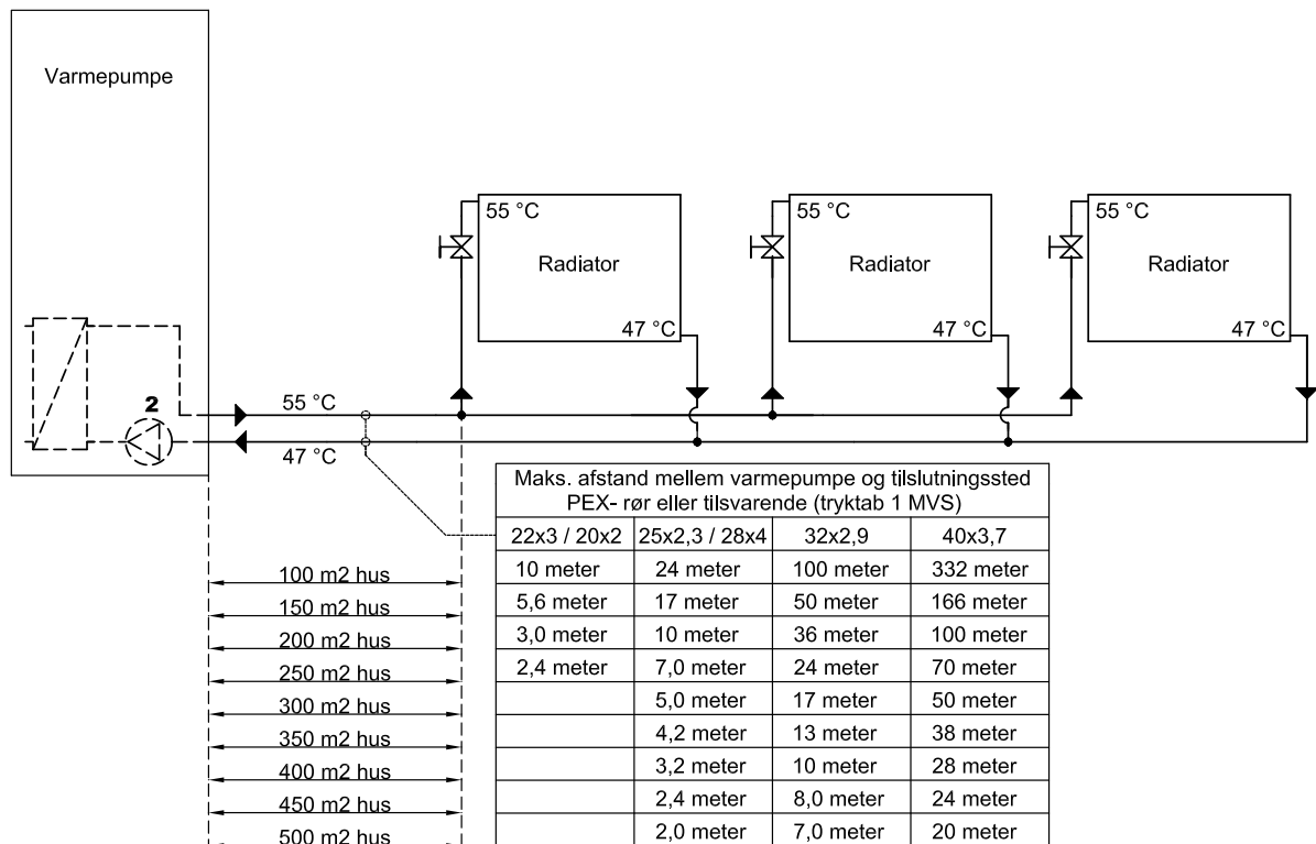
Radiatorer tilkoblet varmpumpe. Temperaturer °C ved vinterdrift.
